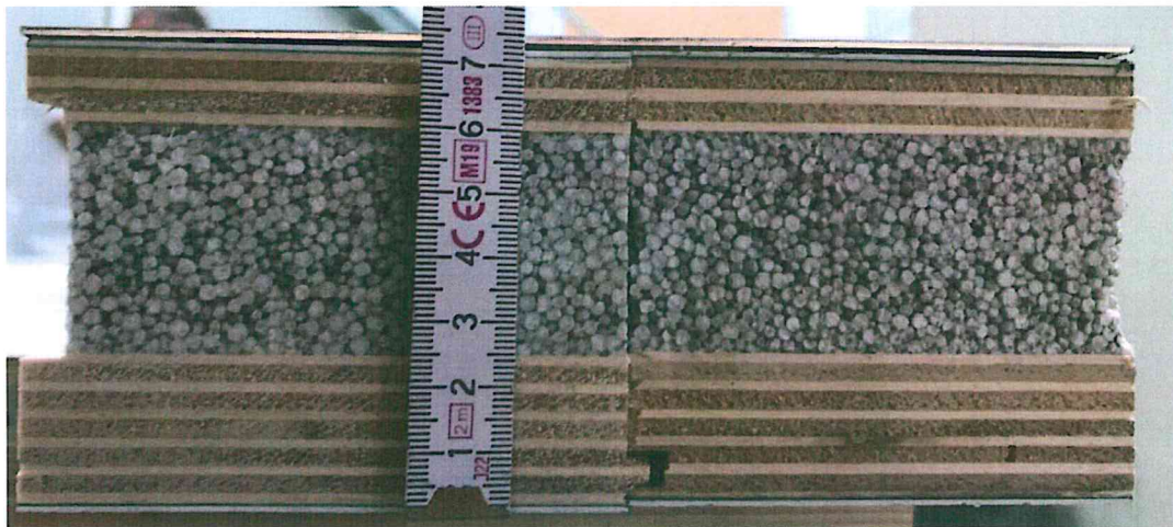
Bild A.3.1: Profilansicht der geprüften Platte
