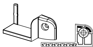
Koncový kryt blaugelb MD V Č. v.řr. 0416859
