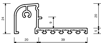
Okapnice blaugelb MD V Č. v.řr. 0416854
