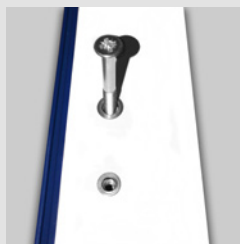
Foto: Element mit Blindnietmuttern zur Befestigung der Rosette
